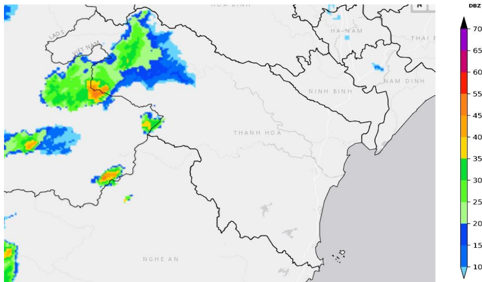
Hình 1: Ảnh radar thời tiết tỉnh Thanh Hoá
