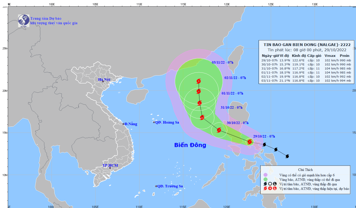
Bản đồ dự báo quỹ đạo và cường độ bão
