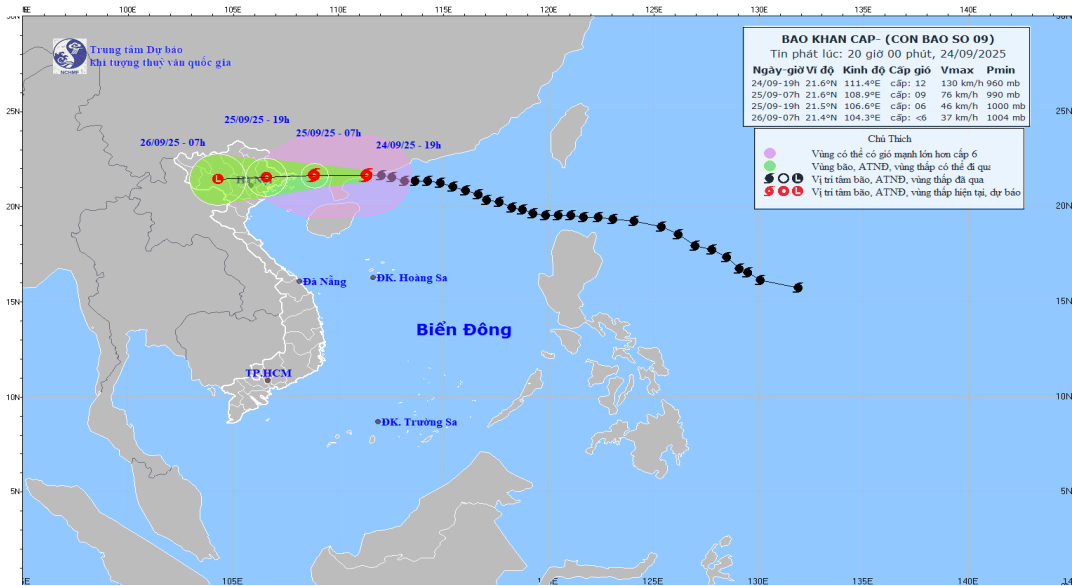
Hình1. Bản đồ dự báo quỹ đạo và cường độ siêu bão số 9 phát lúc 20h00 ngày 24/9/2025 (Nguồn: Trung tâm dự báo KTTV quốc gia)
