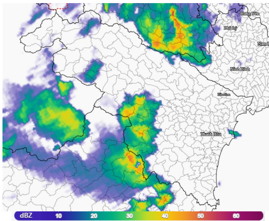
Hình 1: Ảnh radar thời tiết tỉnh Thanh Hoá
