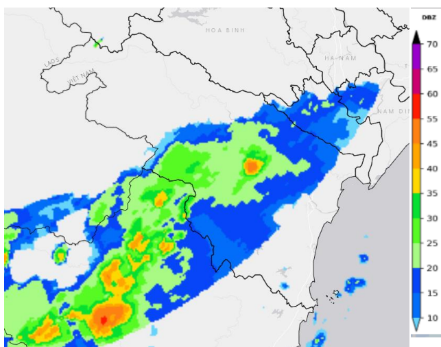
Hình 1: Ảnh radar thời tiết tỉnh Thanh Hoá
