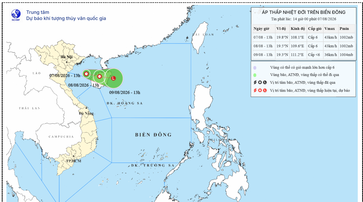
Hình 1. Bản đồ dự báo quỹ đạo và cường độ áp thấp nhiệt đới lúc 14h00 ngày 07/8/2026
